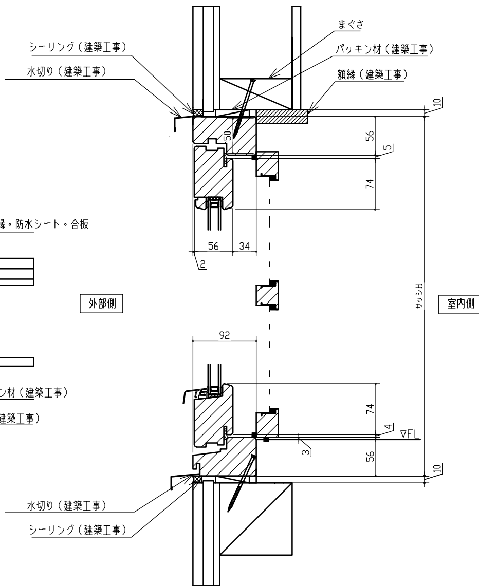
縦断面図
