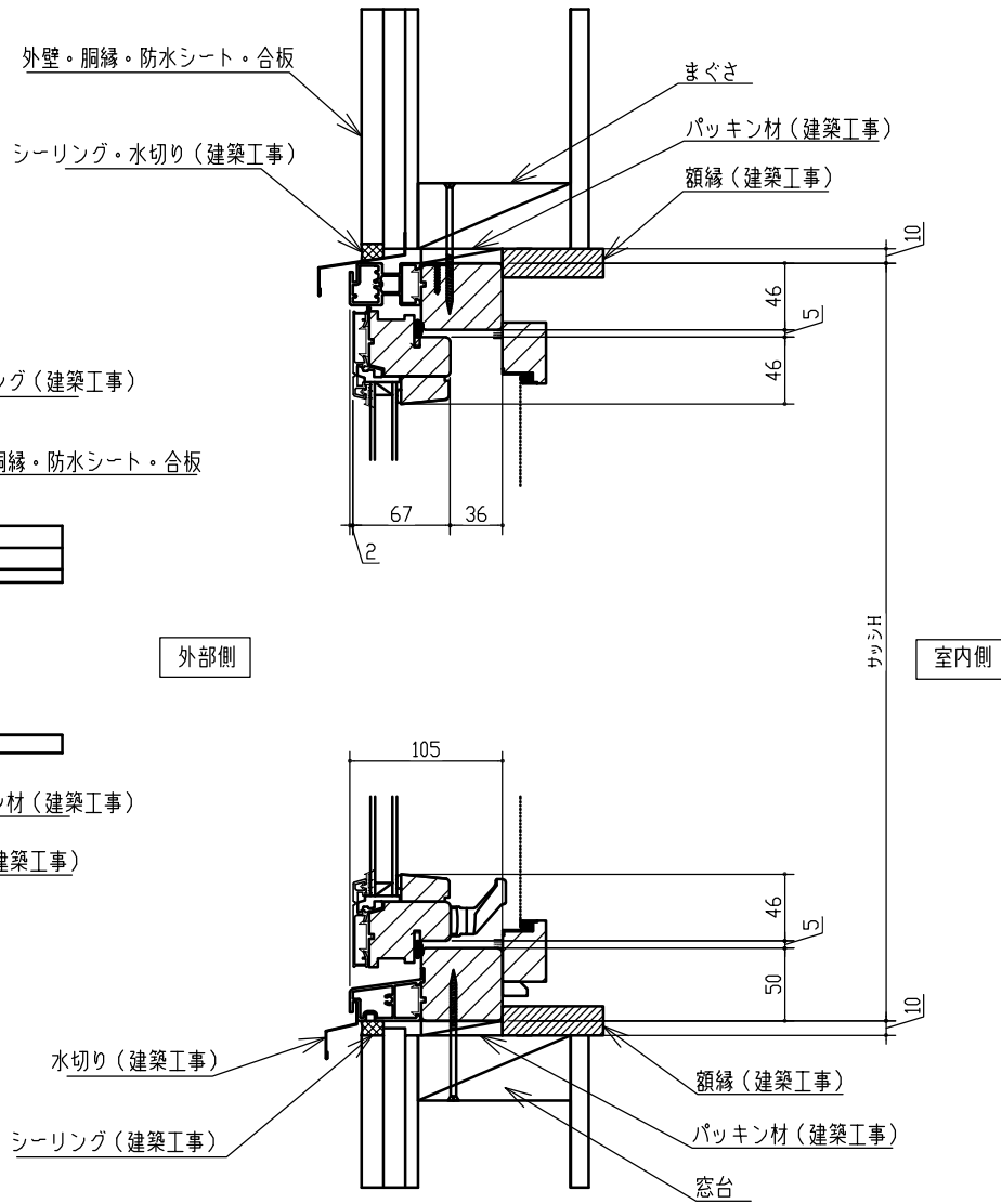
縦断面図
