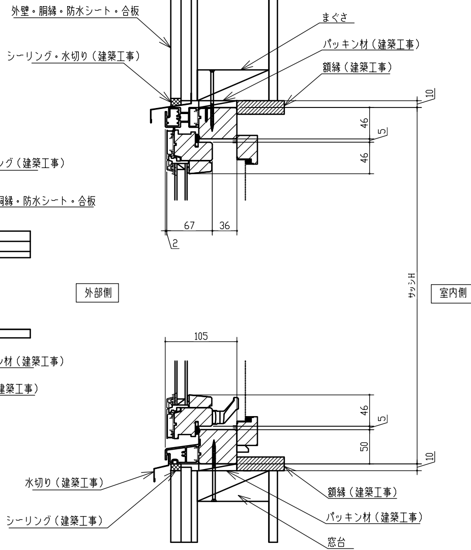
縦断面図
